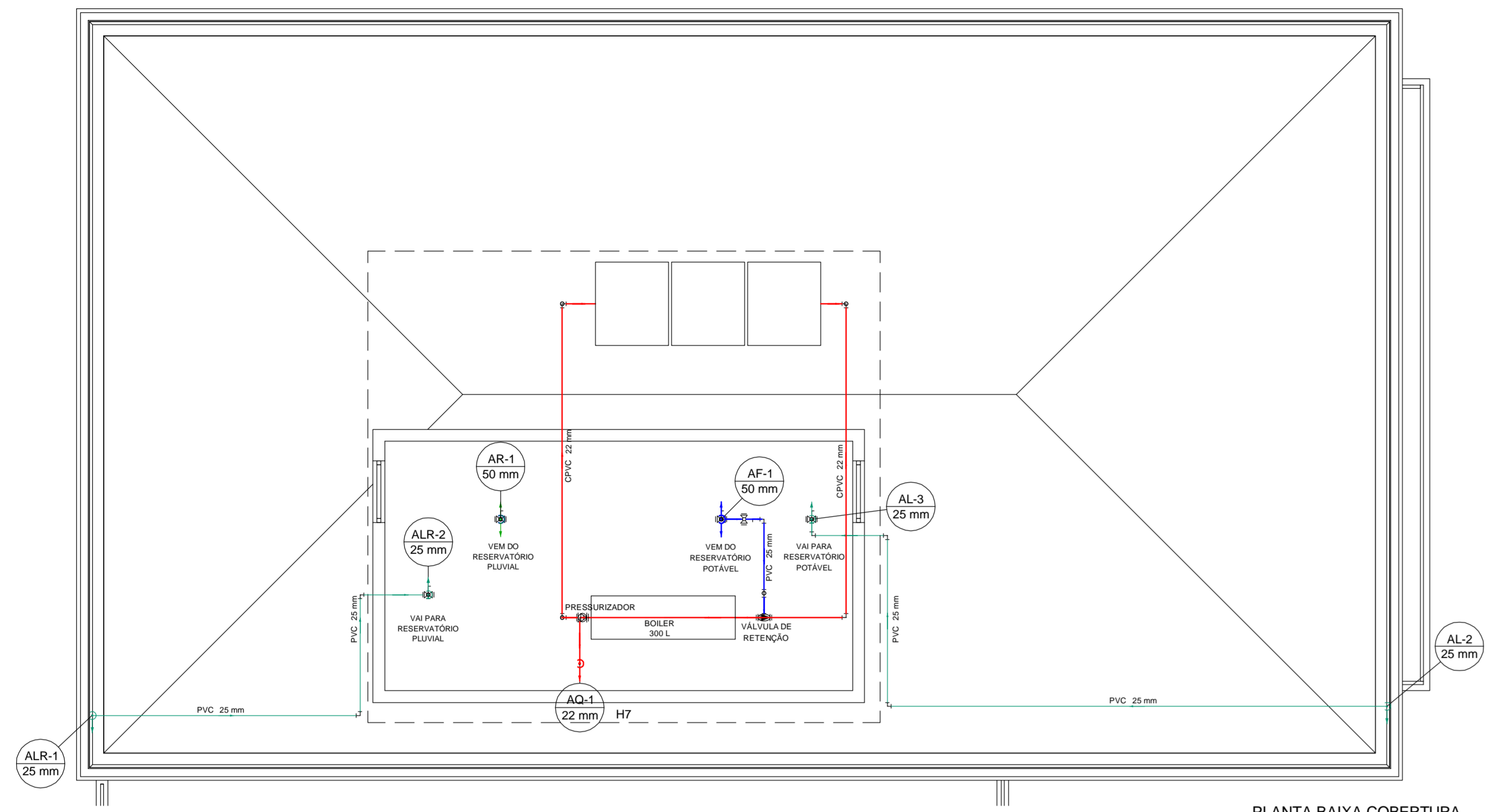
PLANTA BAIXA COBERTURA Esc. 1:50
