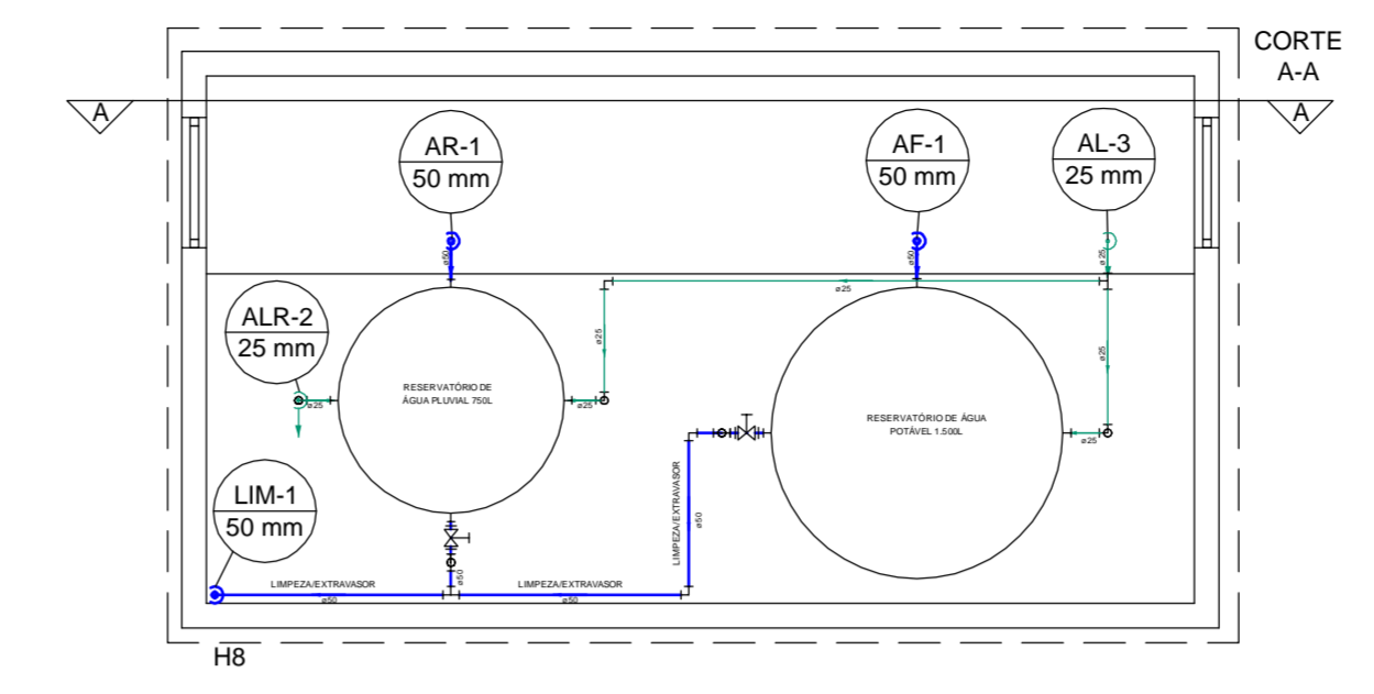
PLANTA BAIXA RESERVATÓRIO Esc. 1:50
