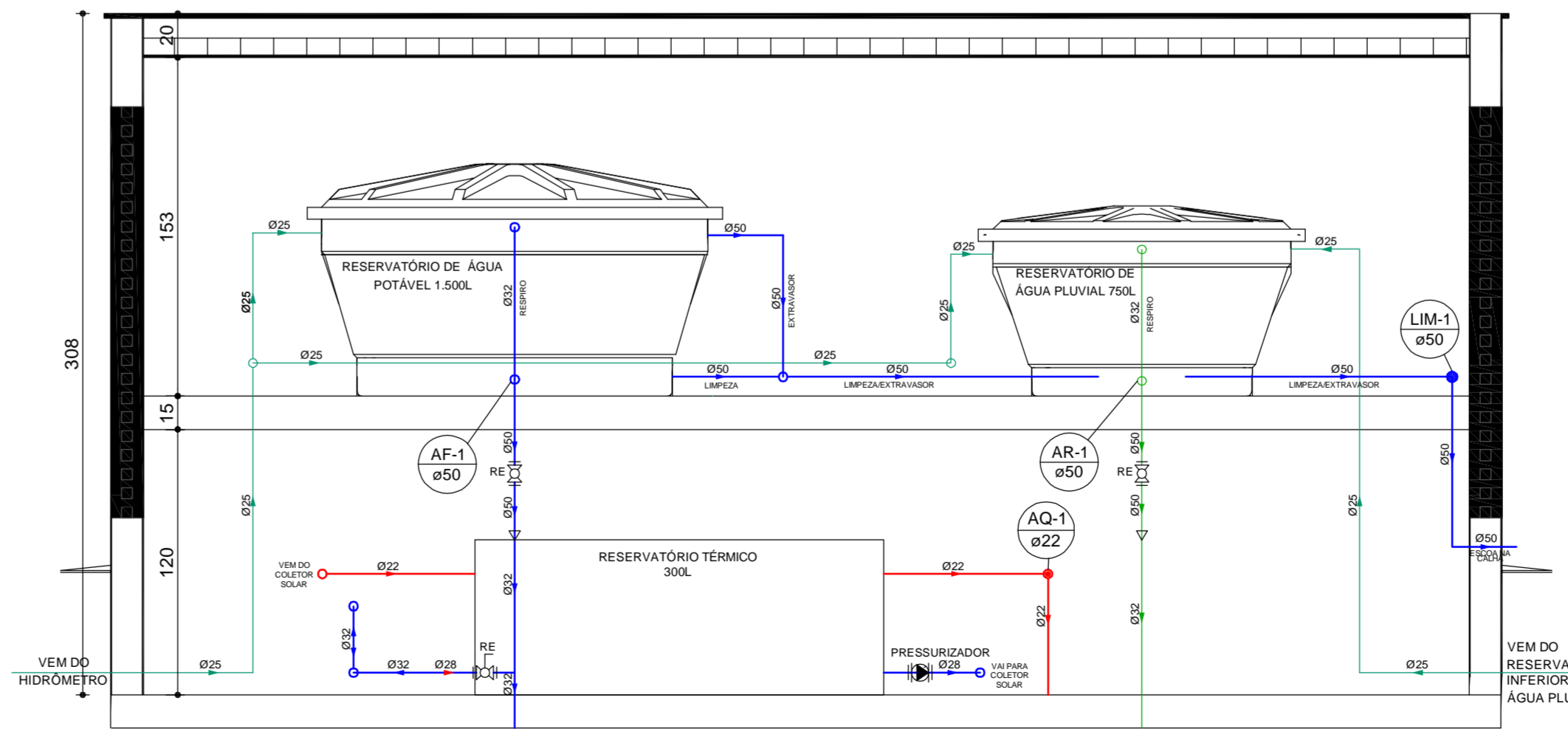
CORTE AA - RESERVATÓRIO ESCALA 1:25
