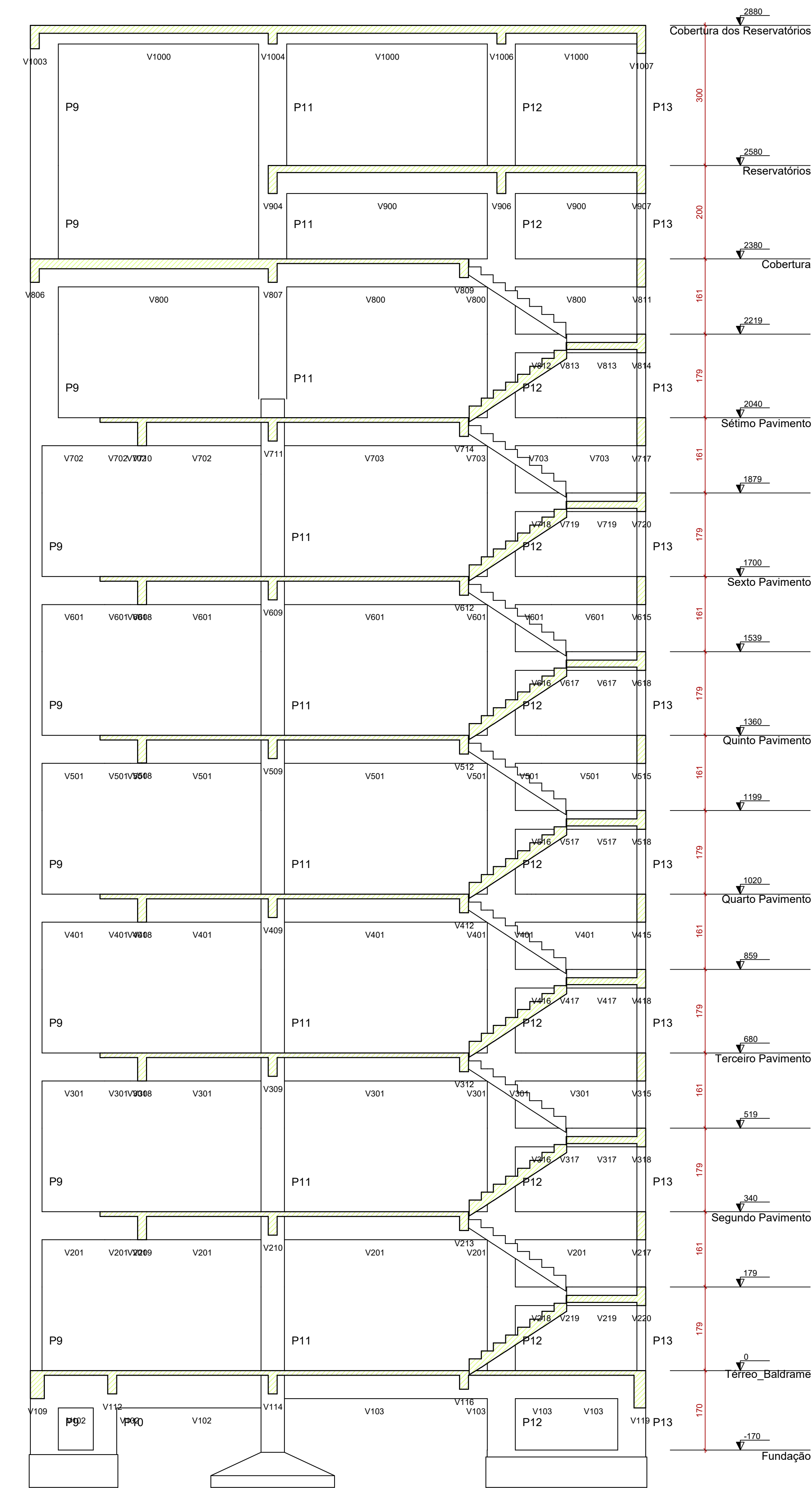
Corte B-B escala 1:60
