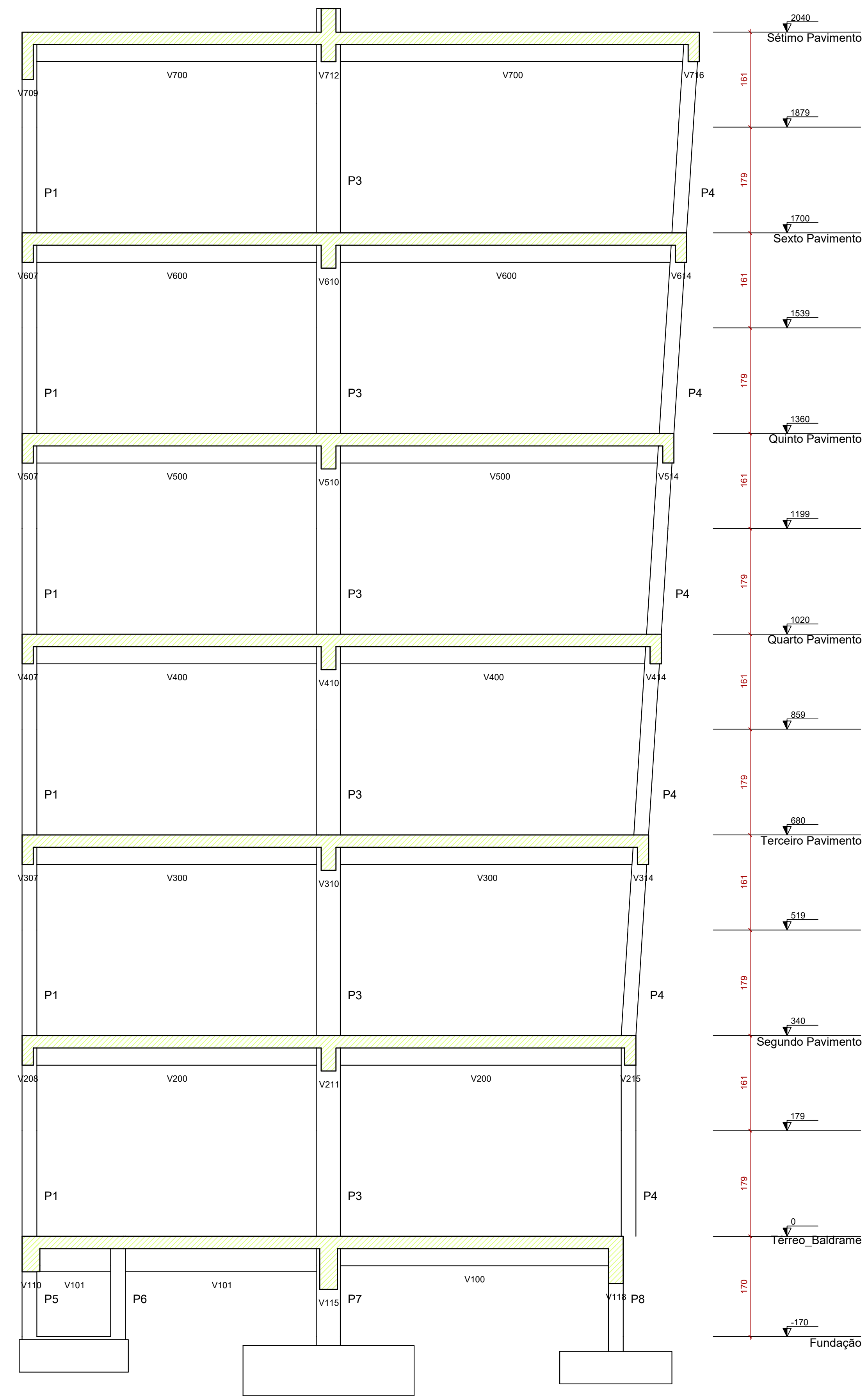
Corte A-A escala 1:50
