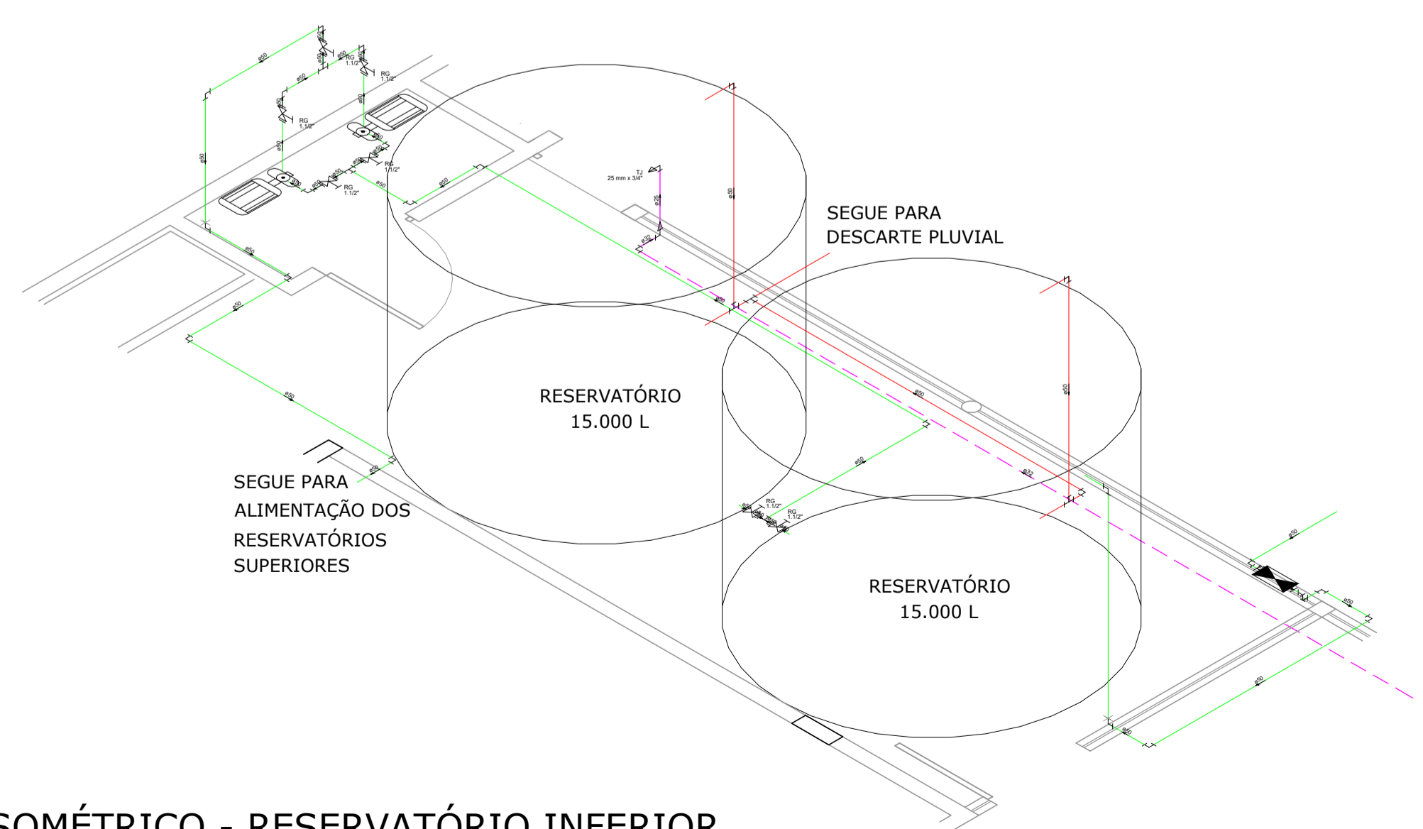
ISOMÉTRICO - RESERVATÓRIO INFERIOR Escala | 1/50
