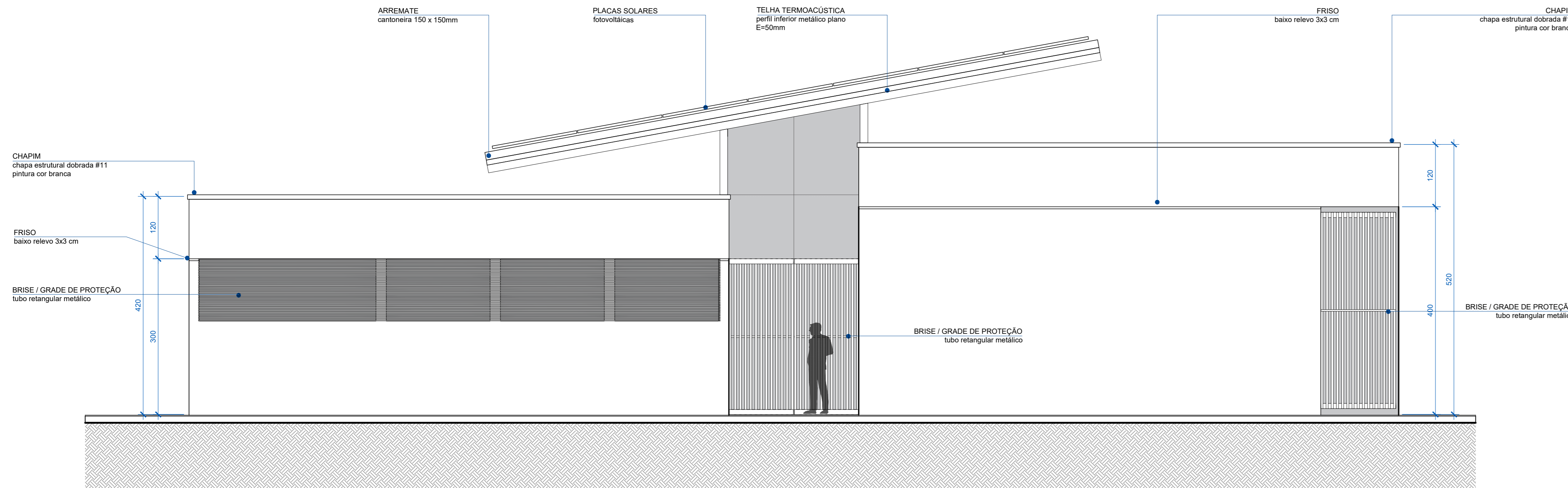
ELEVAÇÃO OESTE ESC 1 : 50
