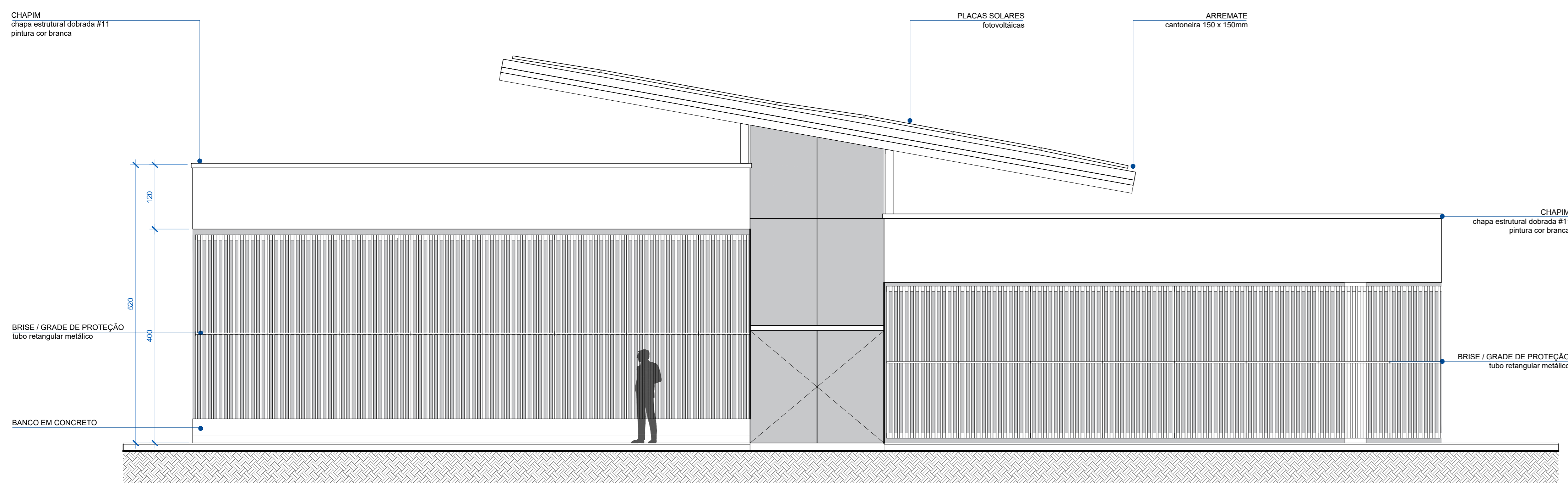
ELEVAÇÃO LESTE ESC 1 : 50
