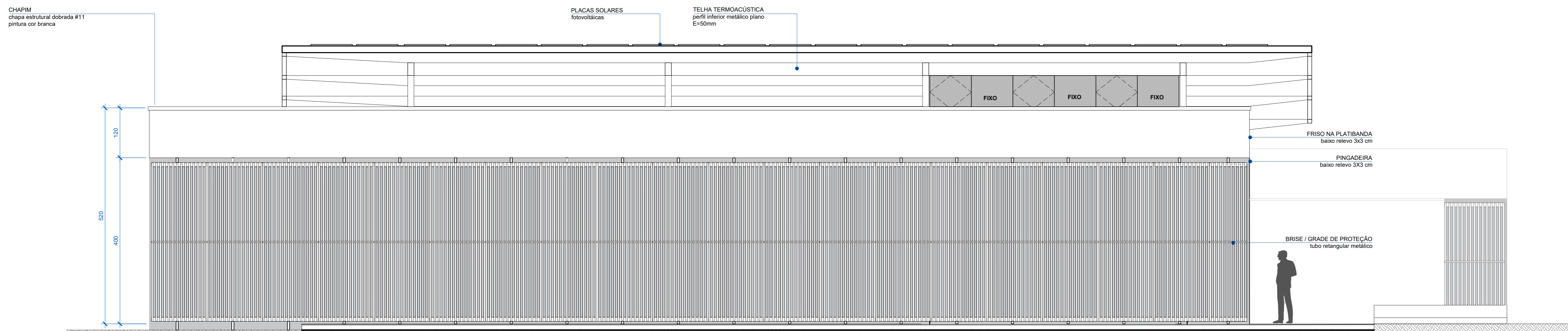
ELEVAÇÃO SUL ESC 1 : 50
