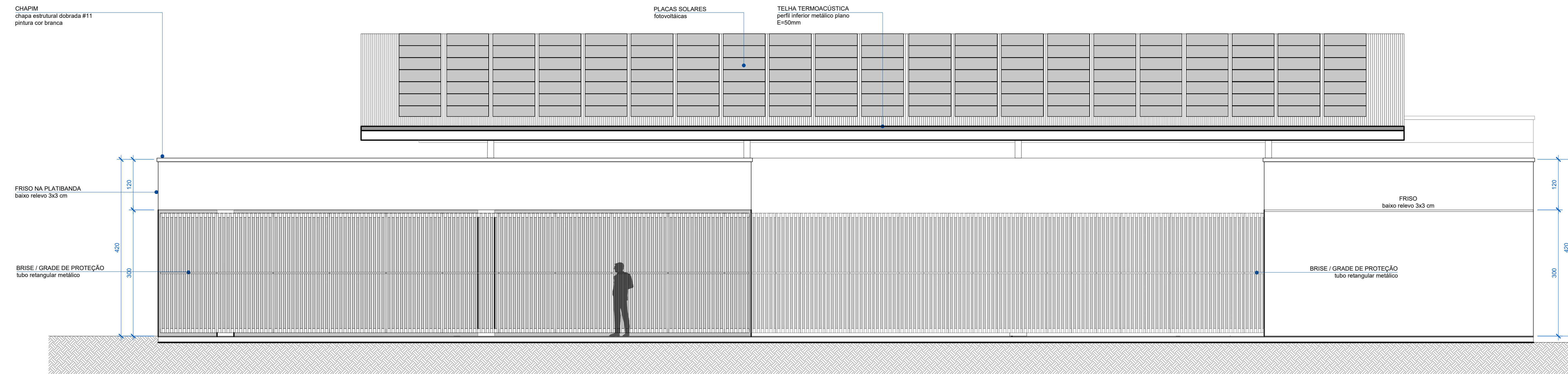
ELEVAÇÃO NORTE ESC 1 : 50
