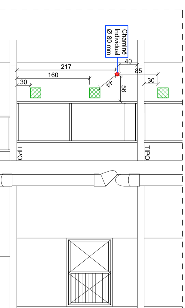
DETALHE SAÍDA DA CHAMINÉ DOS AQUECEDORES
